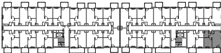
RZUT 1 PIĘTRA, BUDYNEK B
