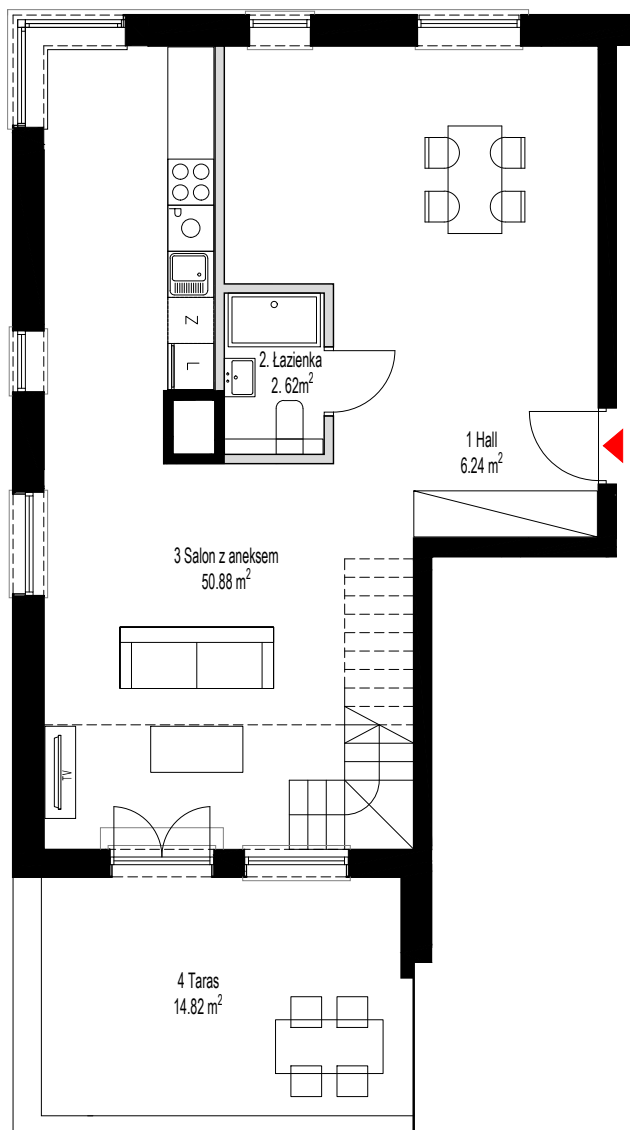
RZUT MIESZKANIA PIĘTRO 3
