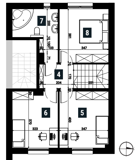
Rzut piętra
