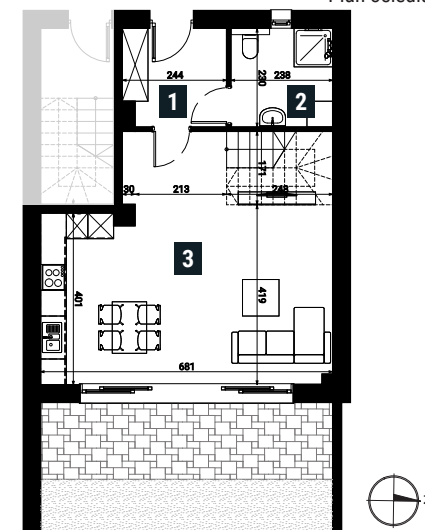
Rzut parteru
