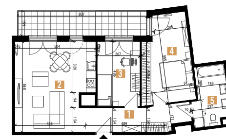
Rzut mieszkania
