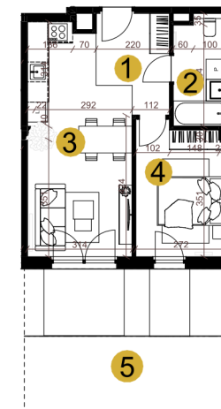
Rzut kondygnacji
