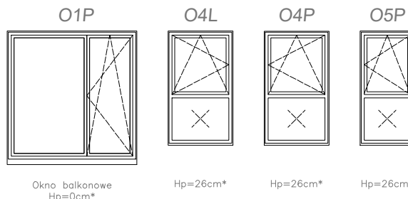
Schemat okien w widoku od wewnątrz:
