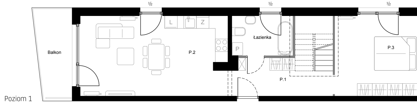
Poziom 1
