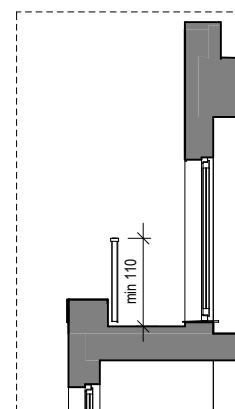
Przekrój przez taras
