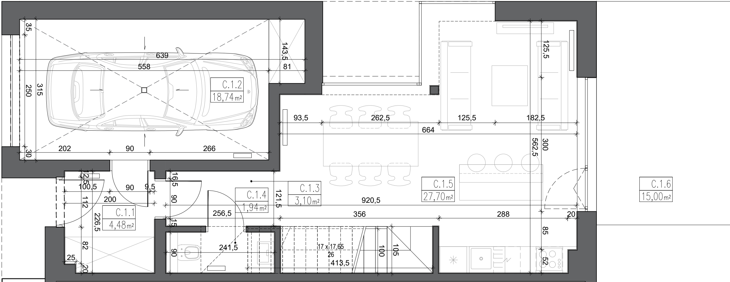
KONDYGNACJA: PARTER
