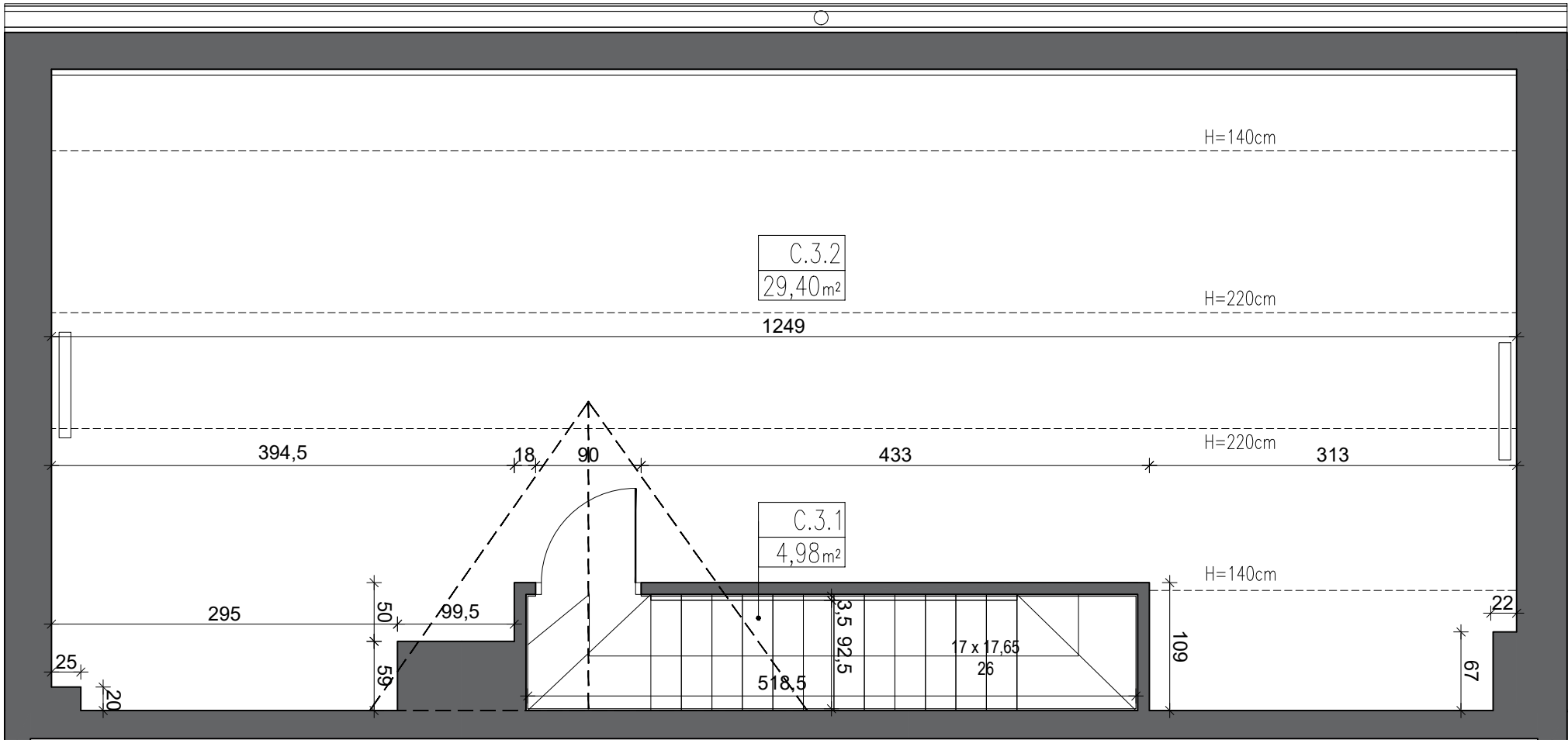
KONDYGNACJA: PODDASZE
