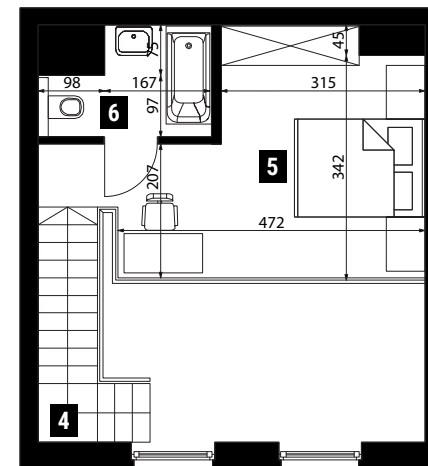
Rzut kondygnacji 2
