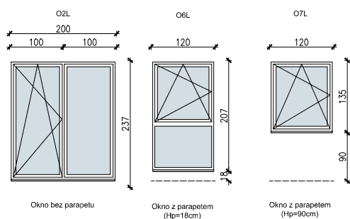
SCHEMAT OKIEN W WIDOKU OD WEWNĄTRZ:
