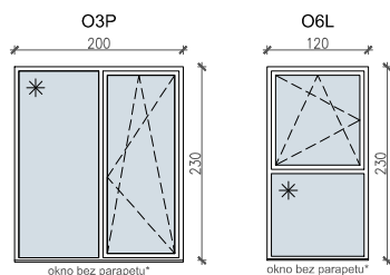
SCHEMAT OKIEN W WIDOKU OD WEWNĄTRZ:
