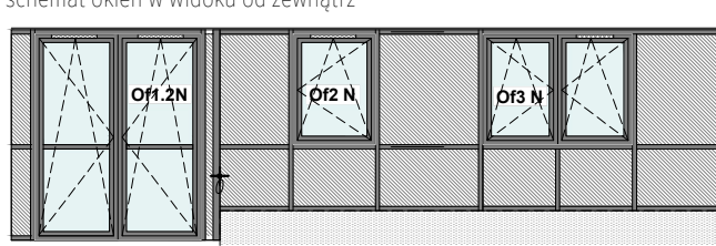
schemat okien w widoku od zewnątrz
