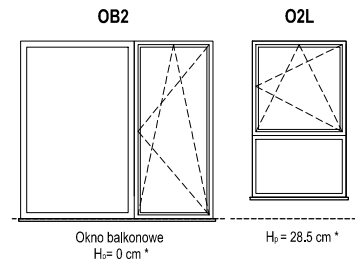
SCHEMAT OKIEN W WIDOKU OD ZEWNĄTRZ
