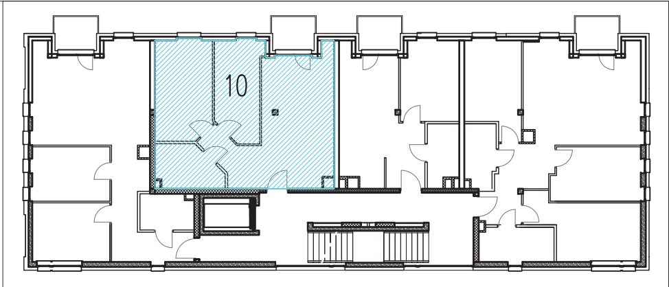
POMIAR POWIERZCHNI LOKALU MIESZKALNEGO Ul. Kartuska 66 – Kondygnacja nr 4, Numer Budowlany 4.M10
