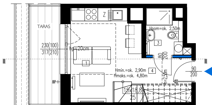
POZIOM 0
