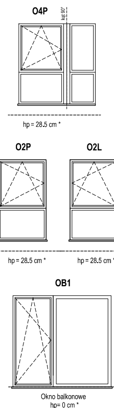
SCHEMAT OKIEN W WIDOKU OD ZEWNĄTRZ
