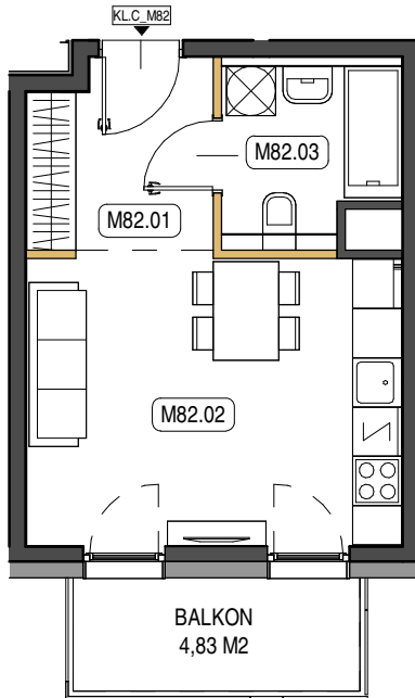
KL.C_M82 - 1 : 100
