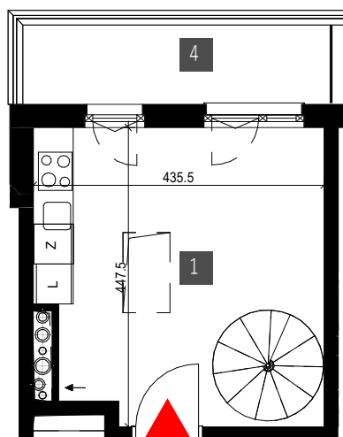
kondygnacja +3
