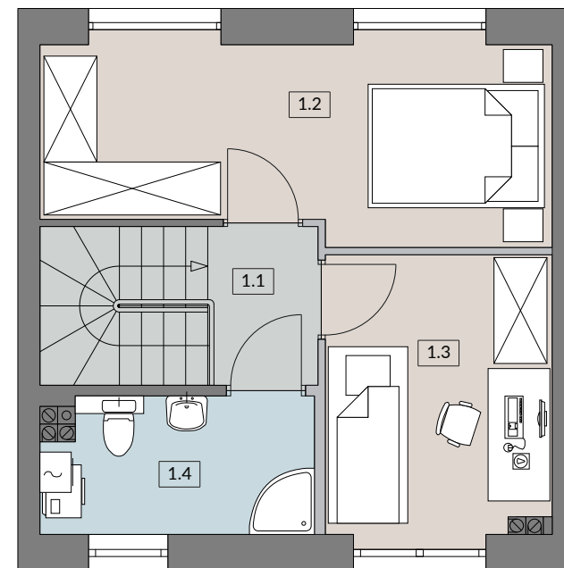
RZUT PIĘTRA
