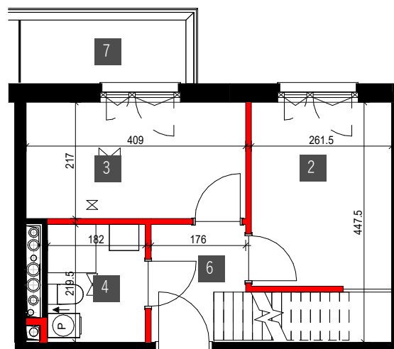
kondygnacja +2
