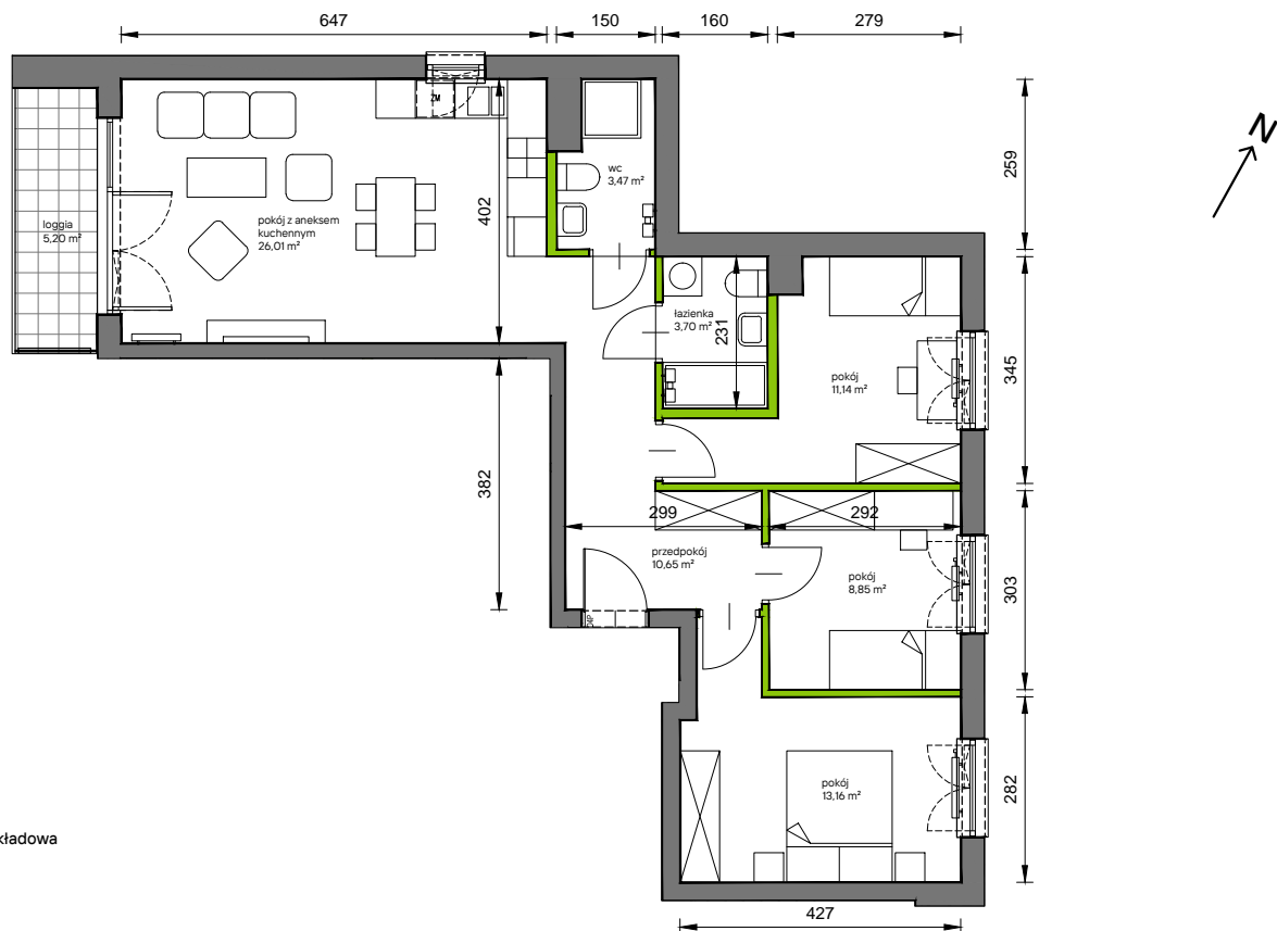
Rzut kondygnacji Piętro 4
