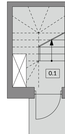
RZUT PARTERU
