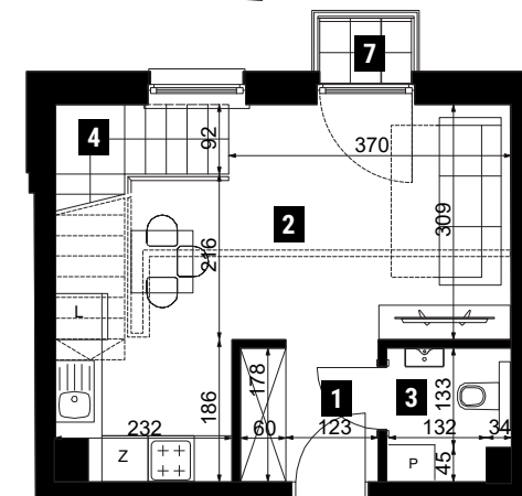
Rzut kondygnacji 7
