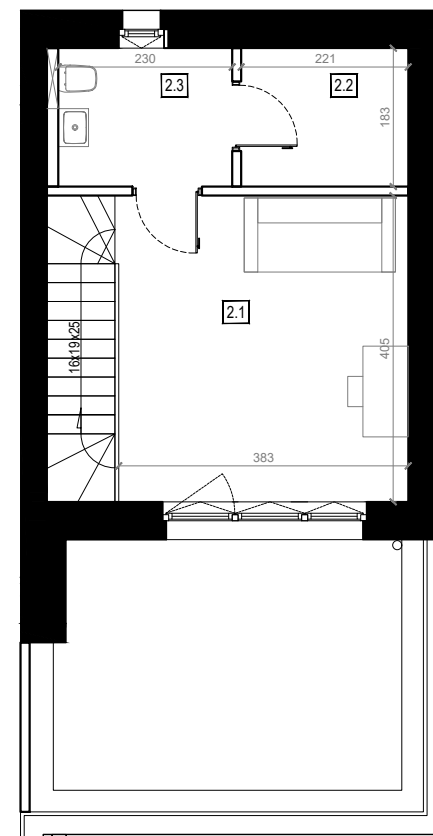
PIĘTRO II
