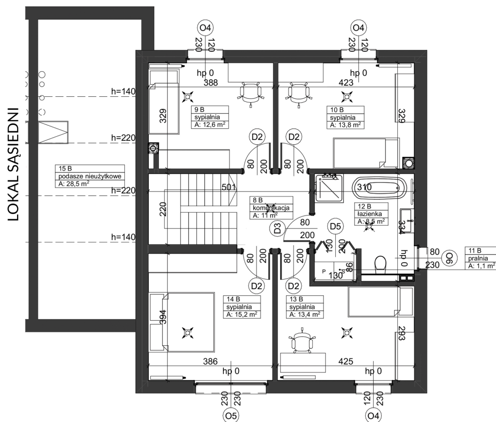
rzut piętra
