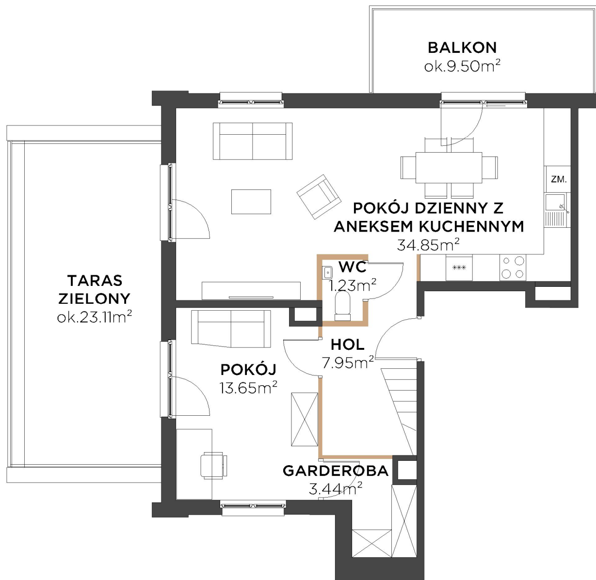
Poziom 1
