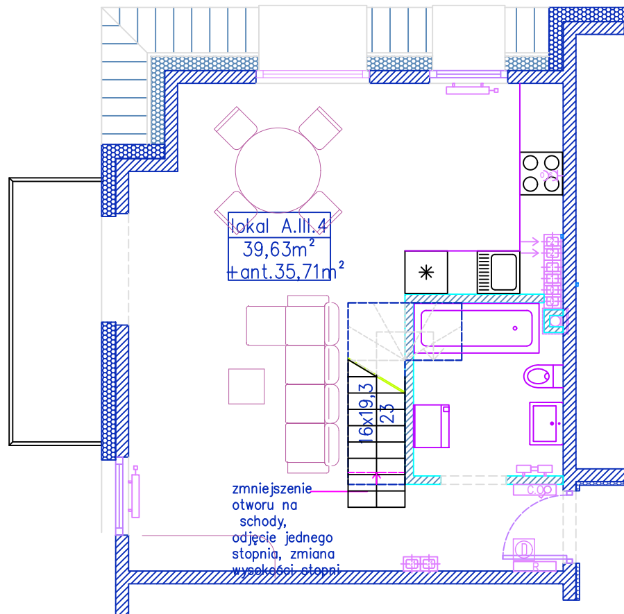
A.III.4 poziom 1
