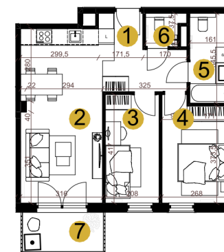
Rzut kondygnacji
