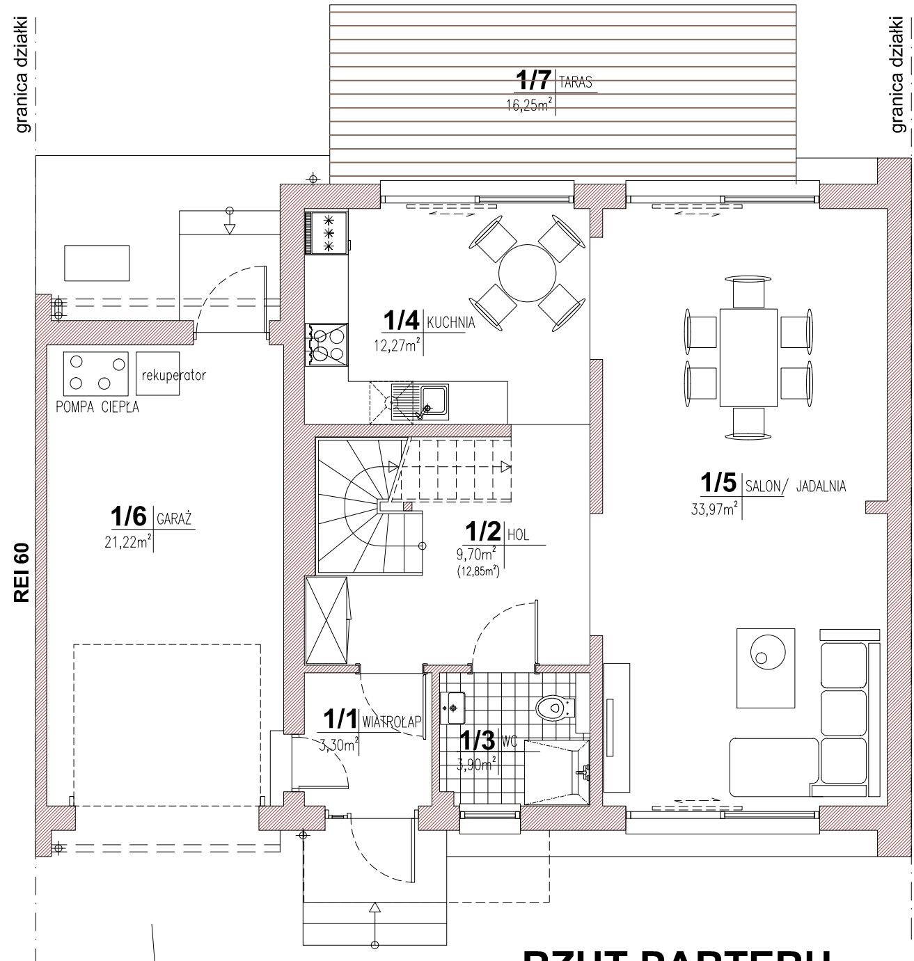
RZUT PARTERU
