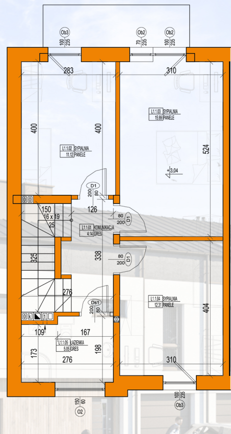
PIĘTRO
