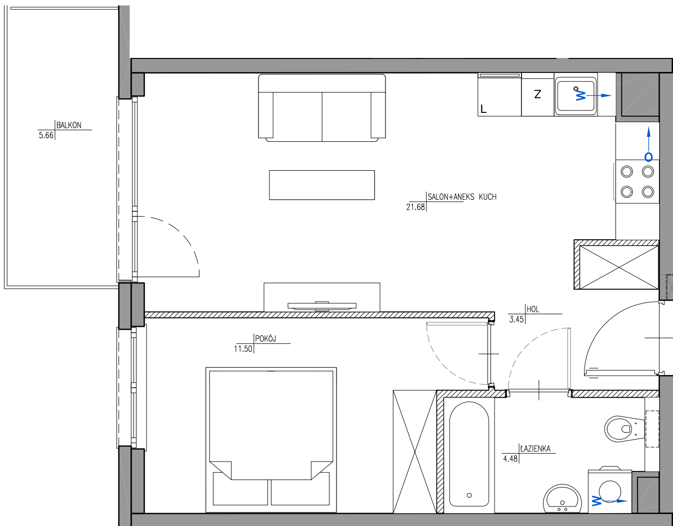
SCHEMAT LOKALU NA RZUCIE
