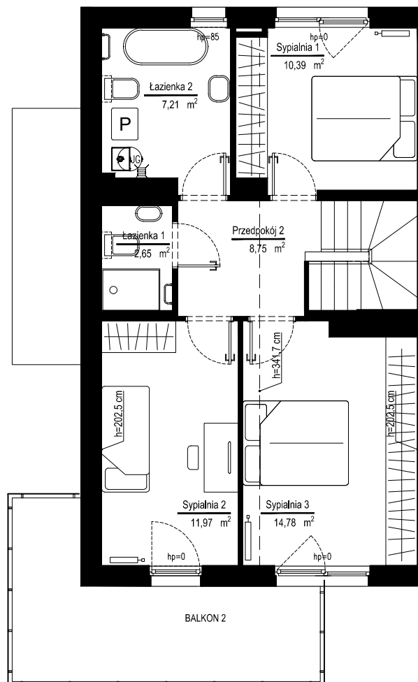
RZUT KONDYGNACJI
