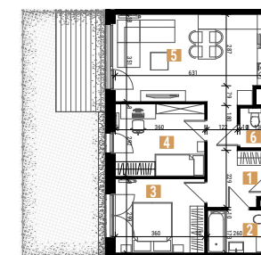
Rzut mieszkania
