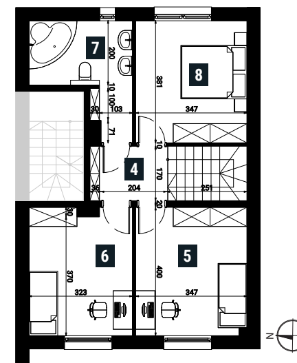
Rzut piętra
