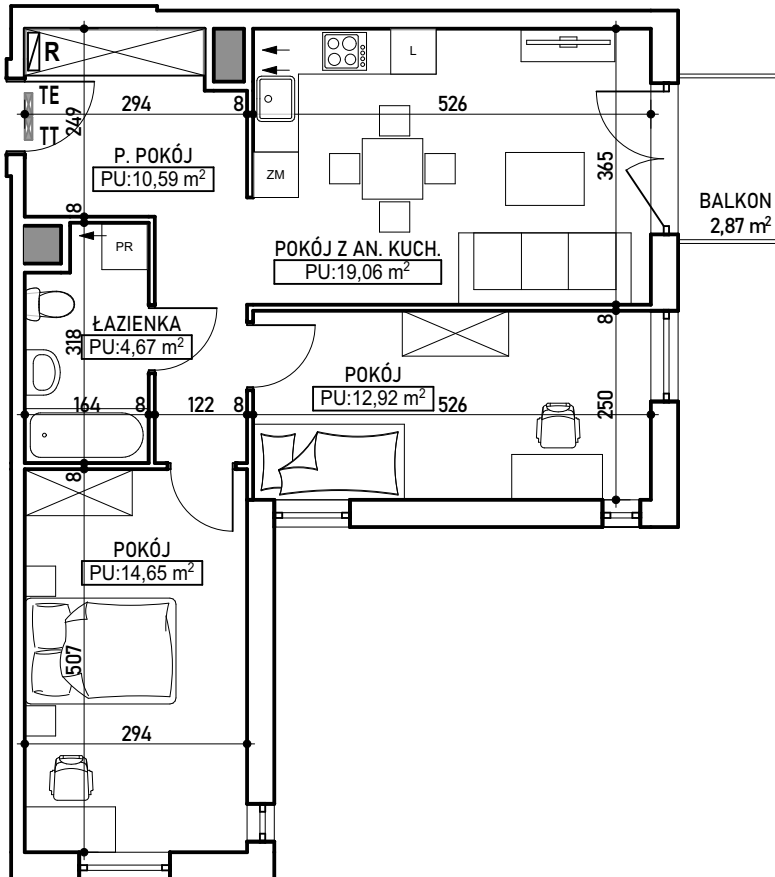
RZUT KONDYGNACJI 4 PIĘTRA BUD. B Z ZAZNACZENIEM LOKALU MIESZKALNEGO
