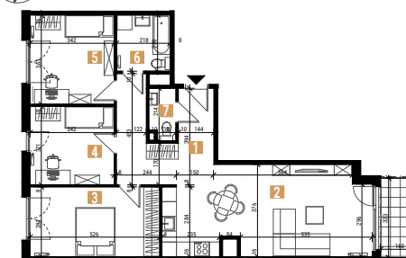
Rzut mieszkania
