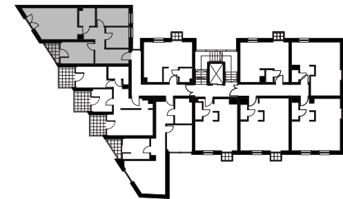
Rzut kondygnacji 5
