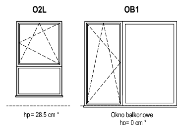
SCHEMAT OKIEN W WIDOKU OD ZEWNĄTRZ
