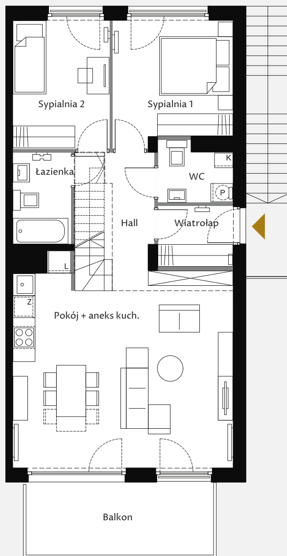
Rzut I piętra
