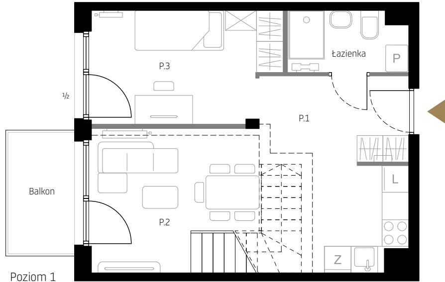
Poziom 1
