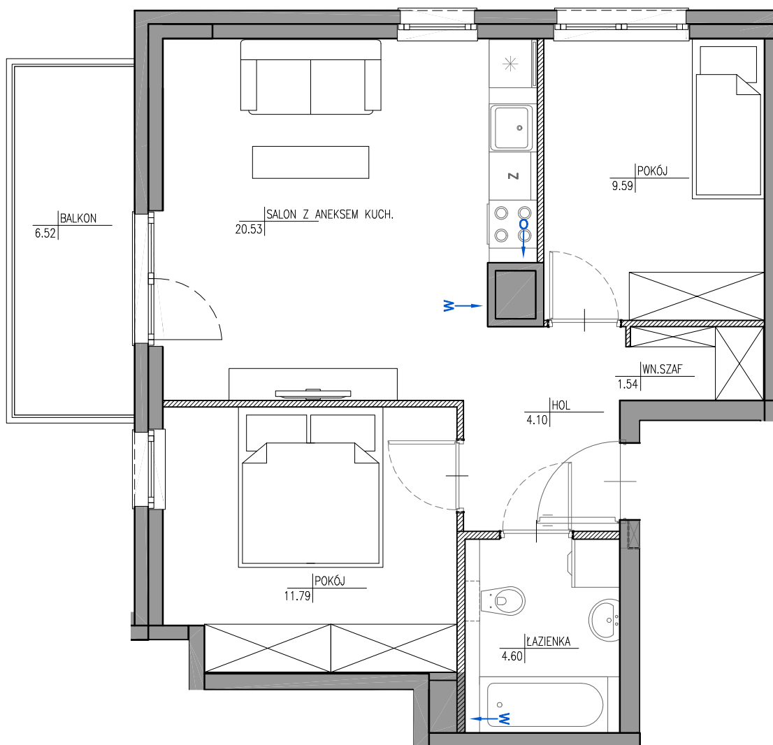
SCHEMAT LOKALU MIESZKALNEGO NA RZUCIE
