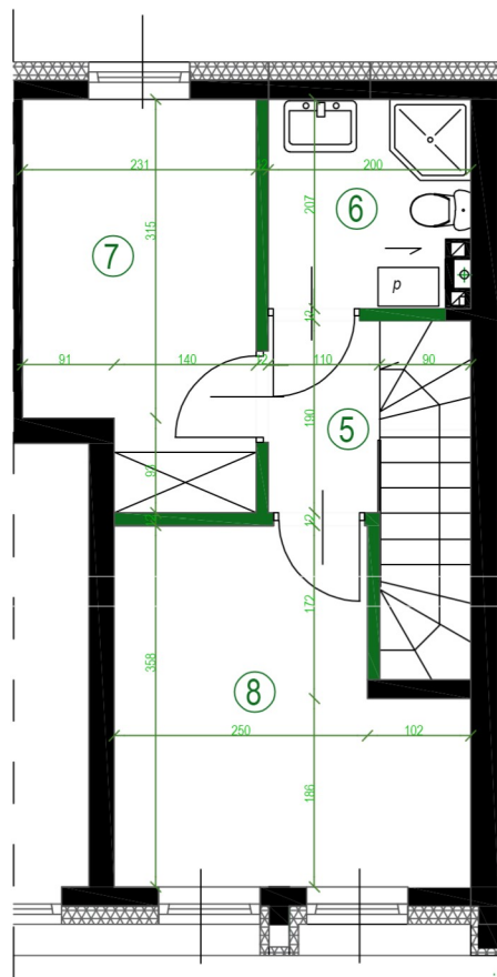
I PIĘTRO
