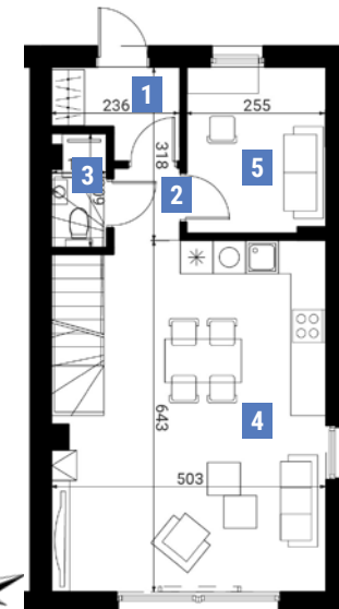
Rzut parteru
