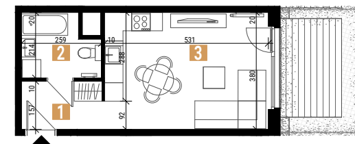
Rzut mieszkania
