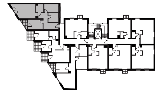
Rzut kondygnacji 3
