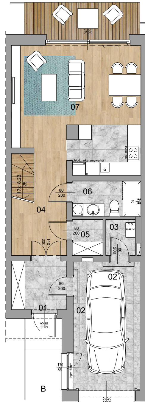
RZUT PARTERU
