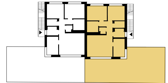
RZUT KONDYGNACJI
