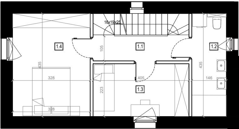
PIĘTRO I
