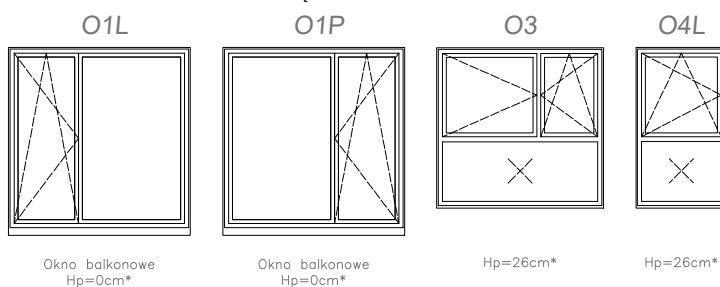
Schemat okien w widoku od wewnątrz:
